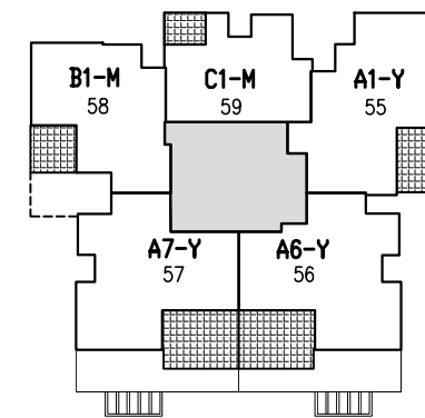
תכנית קומה 12
