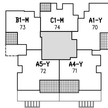
תכנית קומה 15
