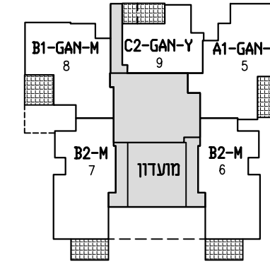
תכנית קומה 2
