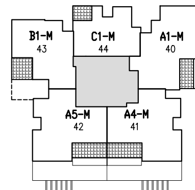
תכנית קומה 9
