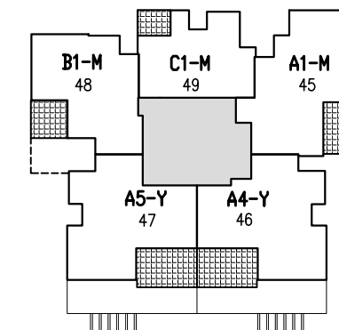
תכנית קומה 10
