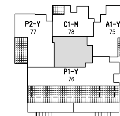
תכנית קומה 16
