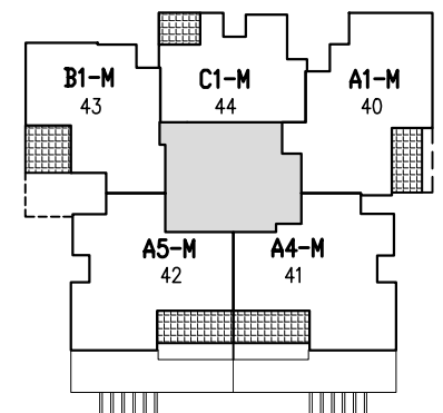
תכנית קומה 9
