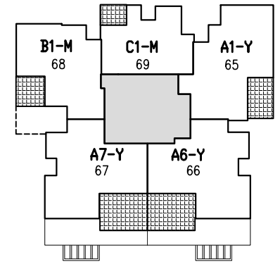
תכנית קומה 14
